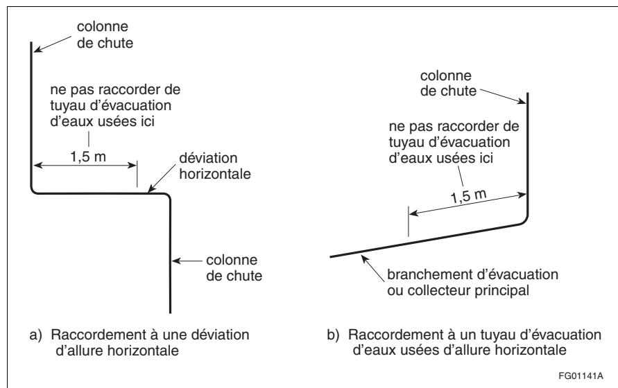
Figure A-2.4.2.1. 2) Raccordements des tuyaux d'évacuation d'eaux usées
