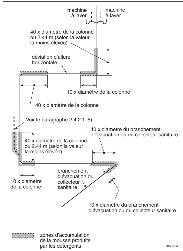
Figure A-2.4.2.1. 4) Zones de pression produites par la mousse
