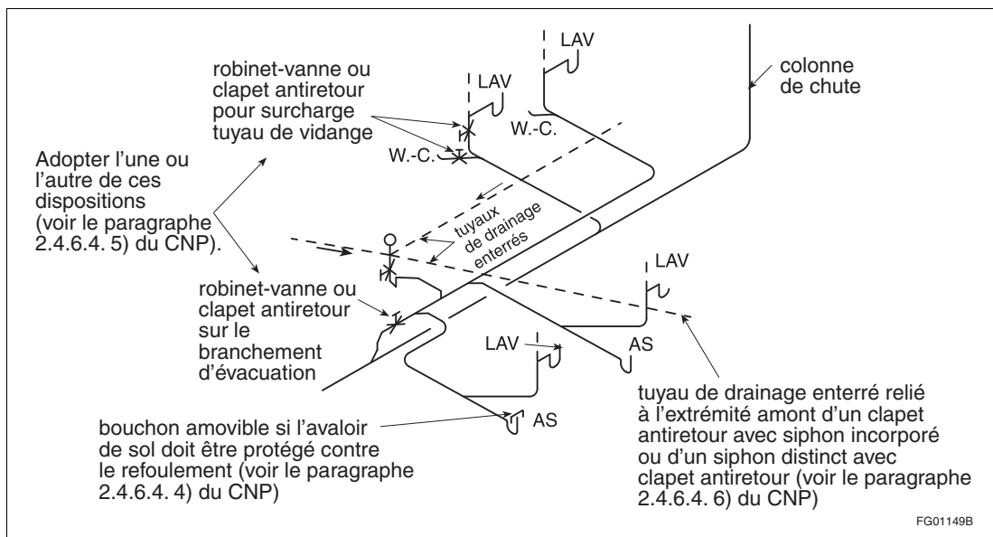
Figure A-2.4.6.4. 6) Protection contre le refoulement causé par une surcharge
