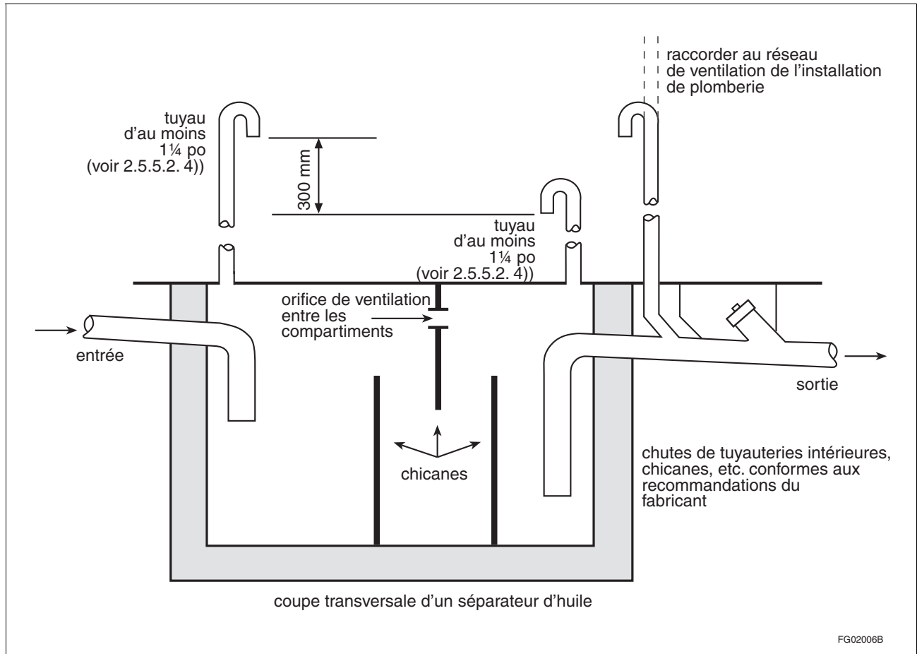
Figure A-2.5.5.2. Séparateurs d'huile
