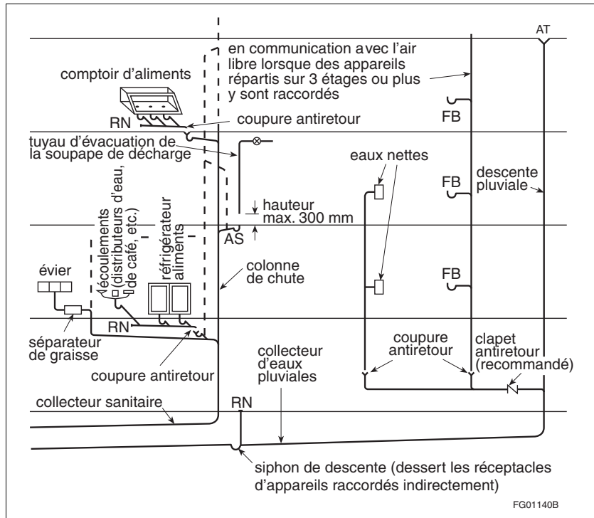
Figure A-2.4.2.1. 1)a)ii) et e)vi) Raccordements indirects
