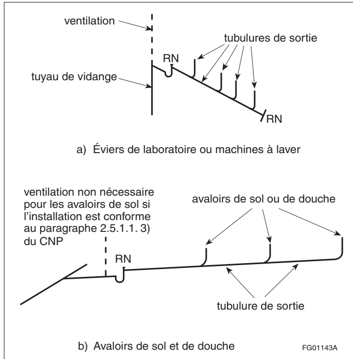
Figure A-2.4.5.1. 3) Siphon unique pour groupe d'appareils
