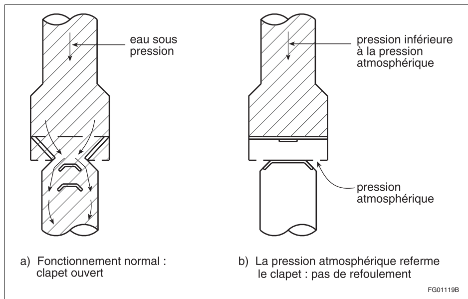
Figure A-1.4.1.2. 1)-B Brise-vide
