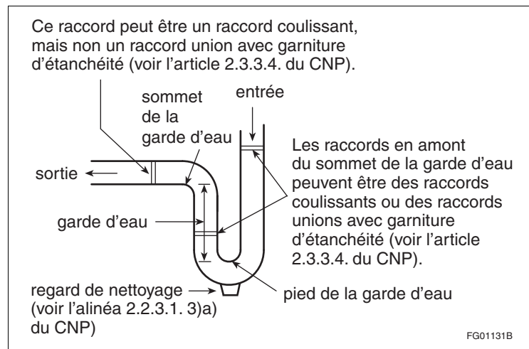
Figure A-2.2.3.1. 1) et 3) Garde d'eau et raccords de siphon
