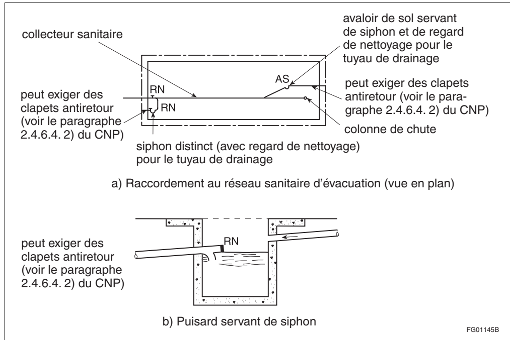
Figure A-2.4.5.3. 1) Raccordement du réseau de drainage
